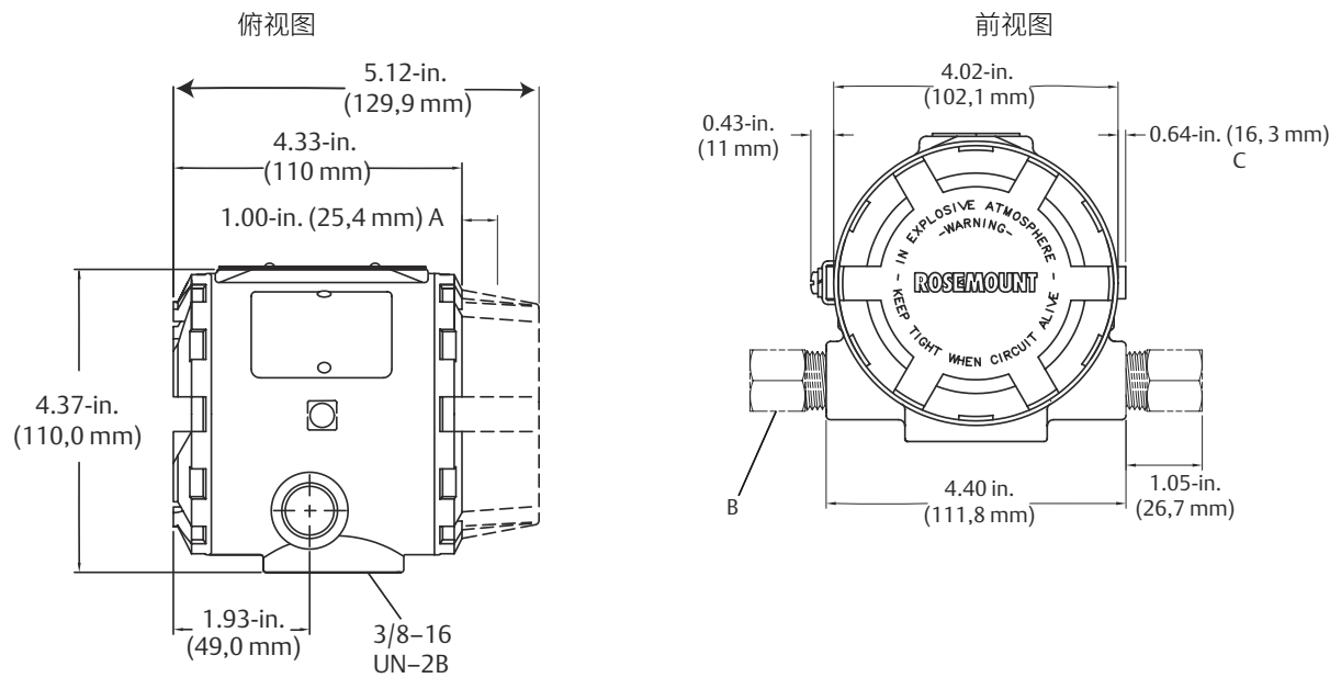
图 5: 适合带有 M20 3 1.5 、 PG 13.5 入口的导线管的变送器
