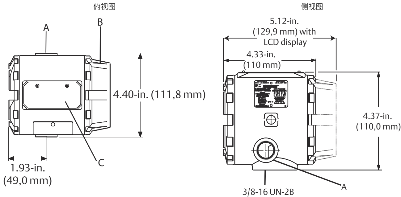
图 4: 变送器视图
